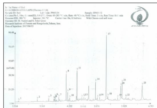
شکل ۱۳: نمودار کروماتوگرام تجزیه اسانس گل‌های جمعیت ۴
